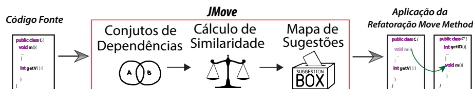
Figure 1. Funcionamento da ferramenta JMove
