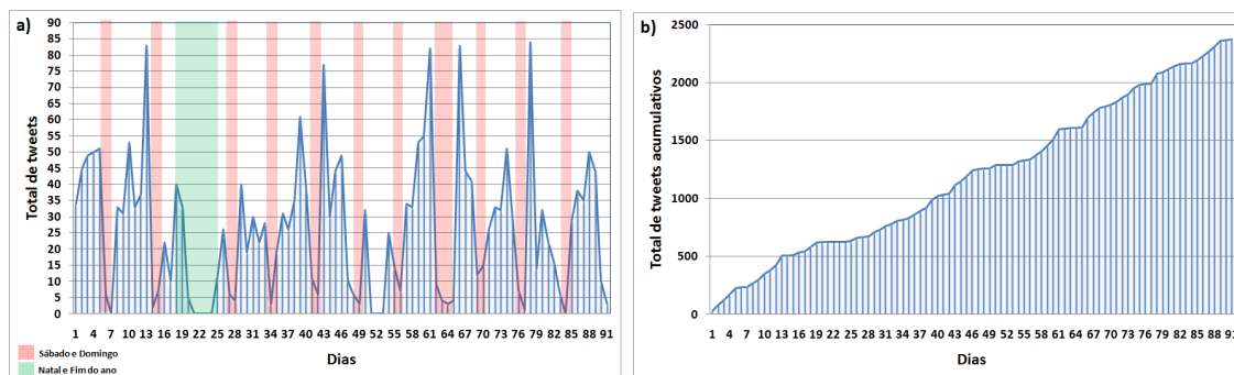
Figura 4. (a) Total de Tweets por Dia (b) Acumulativo de Tweets por Dia
