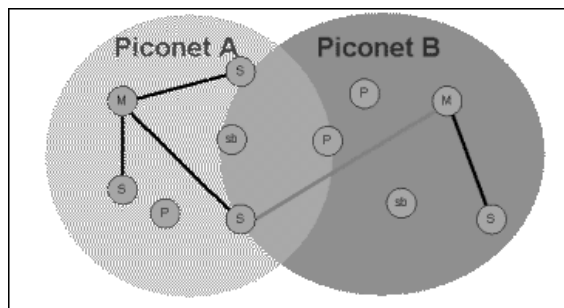
Figura 5.16: Exemplo de piconets formando uma scatternet.
