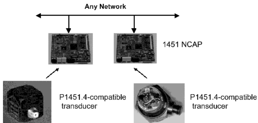
Figura 5.13: Exemplo de interconexão de transdutores (sensores e atuadores usando o padrão IEEE 1451).
