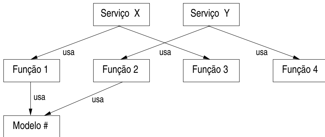
Figura 5.23: Relacionamento entre serviços, funções e modelos.
