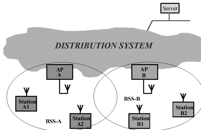
Figura 5.14: Ligação numa rede IEEE 802.11.
