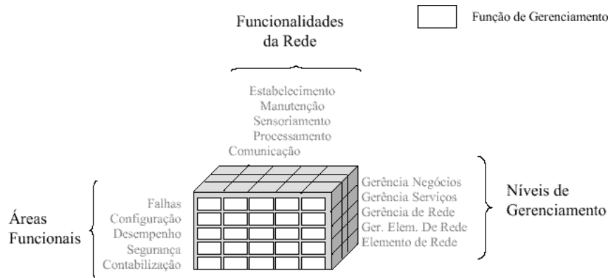
Figura 5.25: Abstrações para as funcionalidades de gerenciamento.
