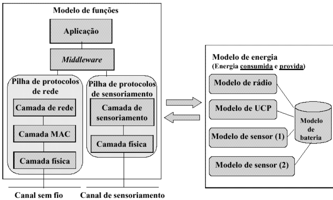
Figura 5.27: Modelo proposto de microsensor do projeto SensorSim.
