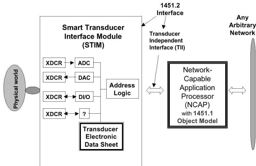
Figura 5.12: Arquitetura do padrão IEEE 1451.
