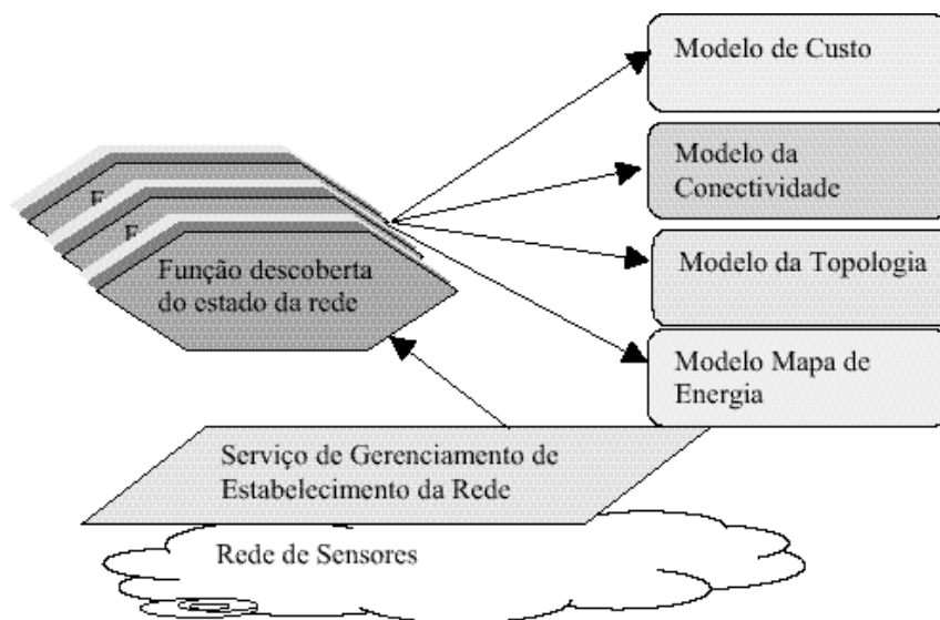
Figura 5.24: Exemplo do relacionamento entre serviços, funções e modelos.
