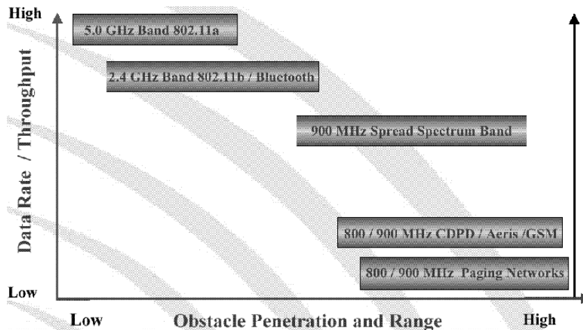
Figura 5.22: Limitações quanto a obstáculos e faixa de alcance.
