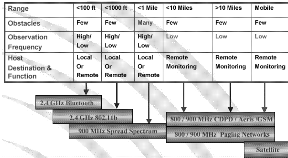
Figura 5.18: Exemplos de tecnologia de comunicação sem fio em função da distância de observação (Fonte Xsilogy).
